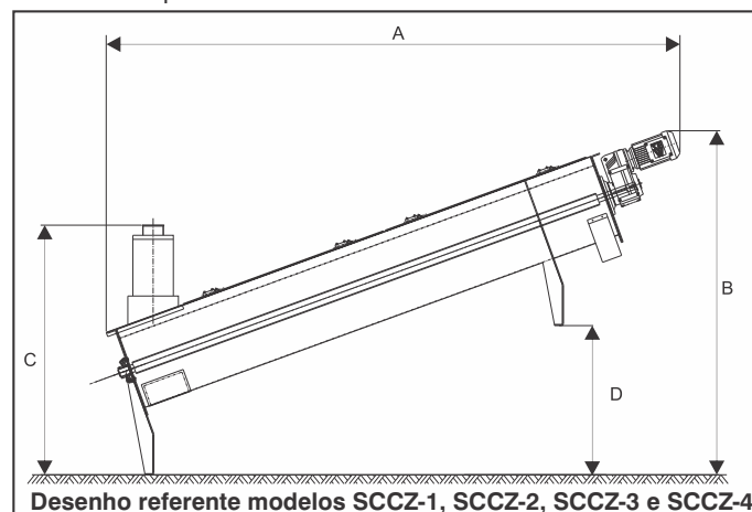
Desenho referente modelos SCCZ-1, SCCZ-2, SCCZ-3 e SCCZ-4
