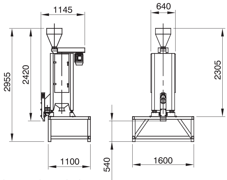
Lay-out con base opcional (dimensiones en mm).
